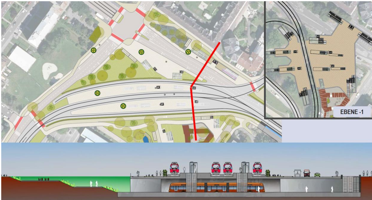
Abbildung 1: Unterirdische Führung der Straßenbahn und oberirdische der Stadtbahn Quelle: ILF
